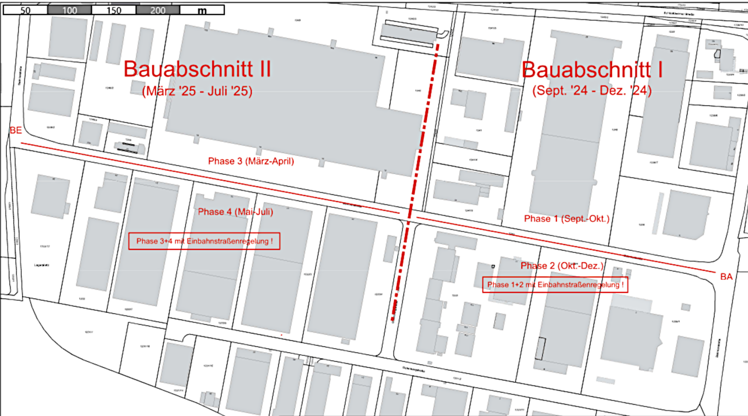
Sanierung Daimlerstraße Übersicht Bauabschnitte/Bauphasen
